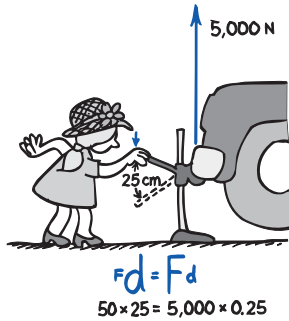
FIGURA 7.14 Fuerza aplicada \times distancia aplicada = fuerza producida \times distancia producida.
