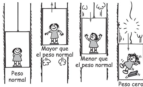
FIGURA 9.9 Tu peso es igual a la fuerza con que comprimes el suelo que te sostiene. Si el suelo acelera hacia arriba o hacia abajo, tu peso varía (aunque la fuerza gravitacional mg que actúa sobre ti permanezca invariable).
