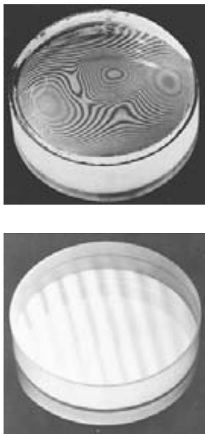
FIGURA 29.24 Planos ópticos para probar qué tan planas son las superficies.
