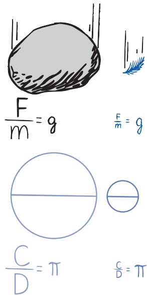
FIGURA 4.13 La relación del cociente entre el peso ( F ) y la masa ( m ) es igual en la piedra grande y en la pluma pequeña; asimismo, la razón entre el perímetro de la circunferencia ( C ) y el diámetro ( D ) es igual para el círculo grande y para el pequeño.
