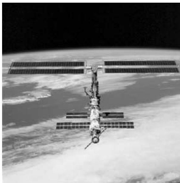
FIGURA 9.11 Los habitantes de esta instalación de laboratorio y puerto experimentan ingravedad continua. Están en caída libre en torno a la Tierra. ¿Actúa sobre ellos alguna fuerza de gravedad?
