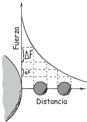
FIGURA 9.15 Gráfica de la gravedad en función de la distancia (no está a escala). Cuanto mayor sea la distancia al Sol, la fuerza F será menor, porque varía según 1/d^2 ; y la diferencia entre atracciones gravitacionales en los lados opuestos de un planeta, \Delta F , es menor, porque varía en función de 1/d^3 y, en consecuencia, las mareas serán menores.
